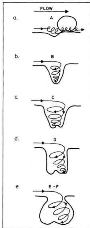
EVOLUCIÓN MORFOLÓGICA DE LAS MARMITAS CON EL TIEMPO
