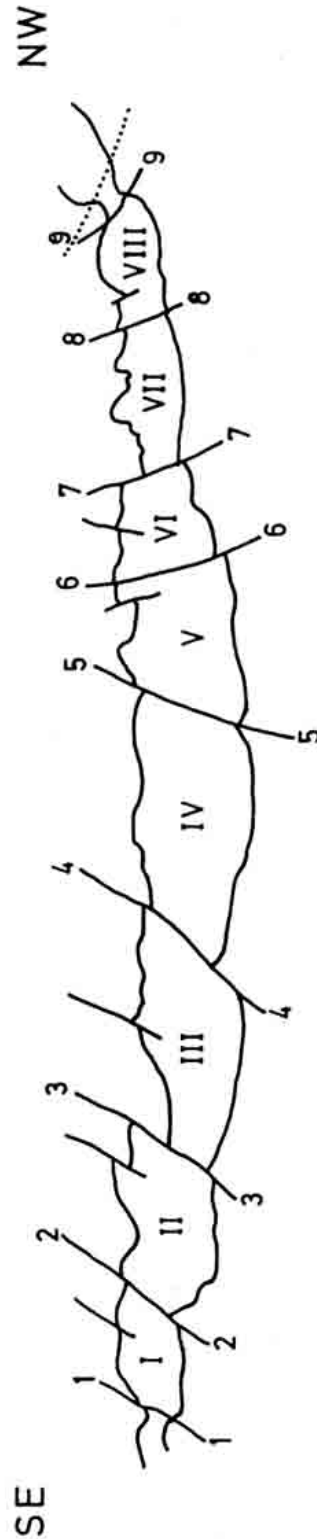
Fig. 2. Esquema, elaborado a partir de fotografías, de ocho pilonos (I-VIII), limitados por nueve fallas notables (1-9). La foto panorámica básica se tomó desde la parte central del valle, por lo que hay una cierta deformación y acortamiento por la perspectiva. Longitud del valle, 120-150 m.; diámetro de las marmitas o pilonos, 10-15 m.
